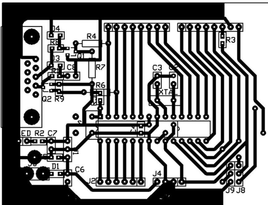
Fig. 2 Schema cablajului imprimat
