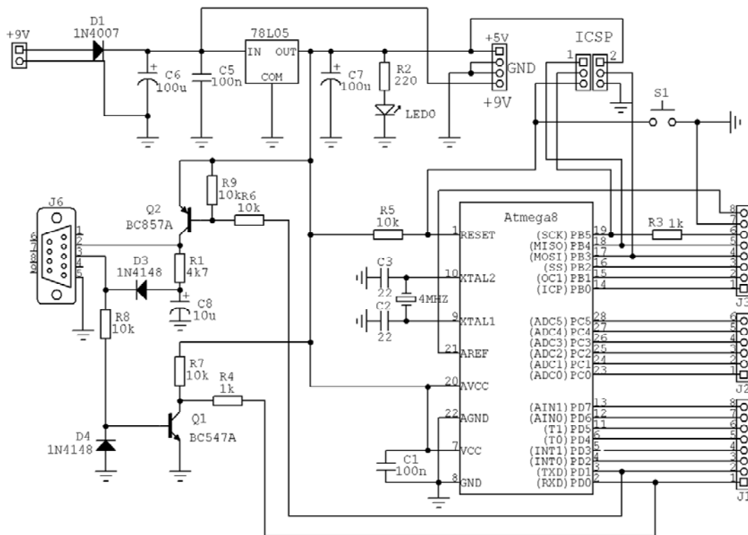
Fig.1 Schema de principiu a kitului de dezvoltare Arduino
